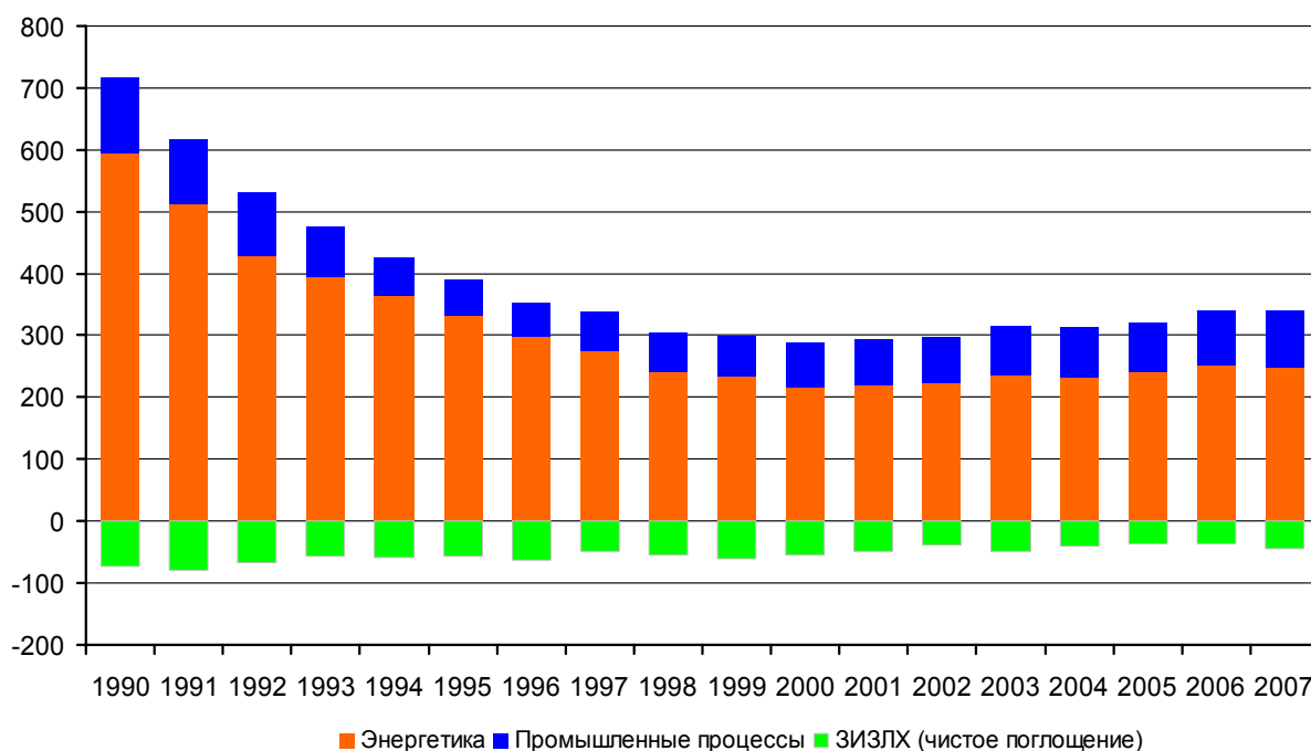
Рис. 3.3. Выбросы и поглощение диоксида углерода в Украине по секторам, 1990-2007 гг., млн. т
