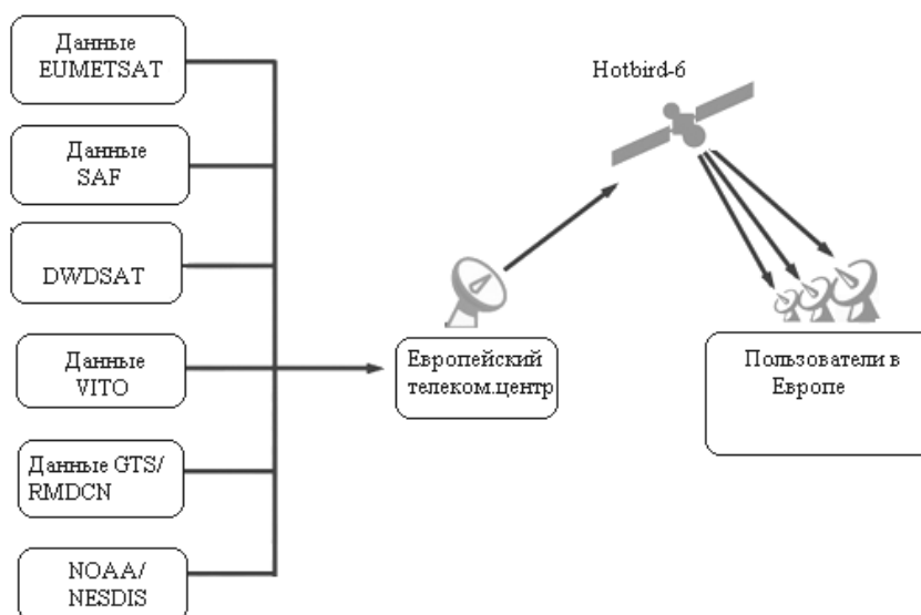
Рис. 8.1. Схема сбора и передачи данных EUMETCast
