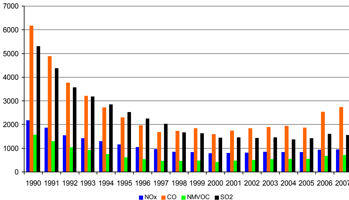
Рис. 3.8. Выбросы ПГ косвенного действия и SO 2 в Украине, 1990-2007 гг., тыс. т
