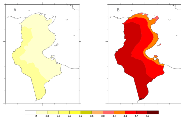
Figure 13 : Evolution de la température moyenne annuelle (en °C) à l'horizon 2050 (A) et à l'horizon 2100 (B) avec le scénario RCP 8.5 (Source : INM)
