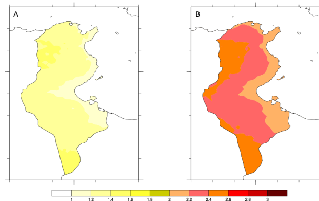
Figure 12 : Evolution de la température moyenne annuelle (en °C) à l'horizon 2050 (A) et à l'horizon 2100 (B) avec le scénario RCP 4.5 (Source : INM)
