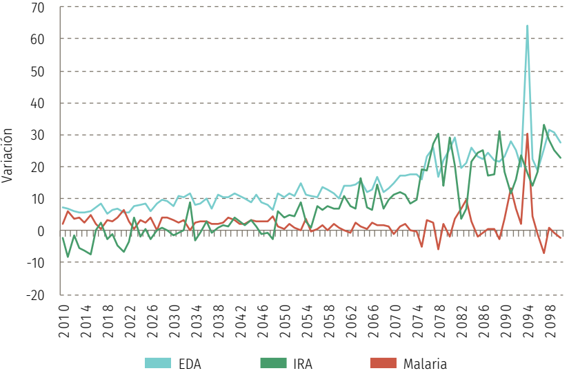
Gráfico 17: Proyecciones en número de casos. EDA, IRA y malaria. Escenario A2
