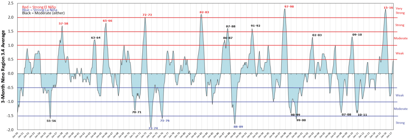
Gráfico 4: Eventos extremos. Inundaciones y sequías históricas periodo 1950-2016
