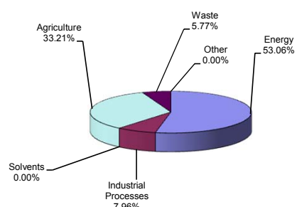
2010
