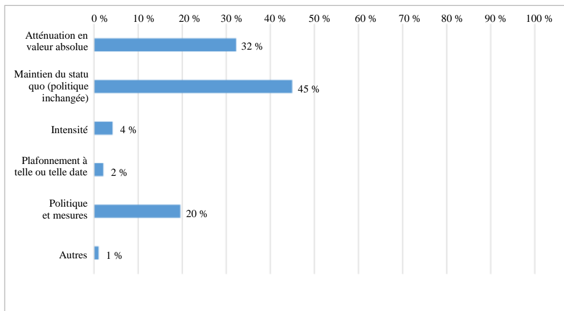
Figure 1 Types d'objectif d'atténuation communiqués dans les contributions prévues déterminées au niveau national
