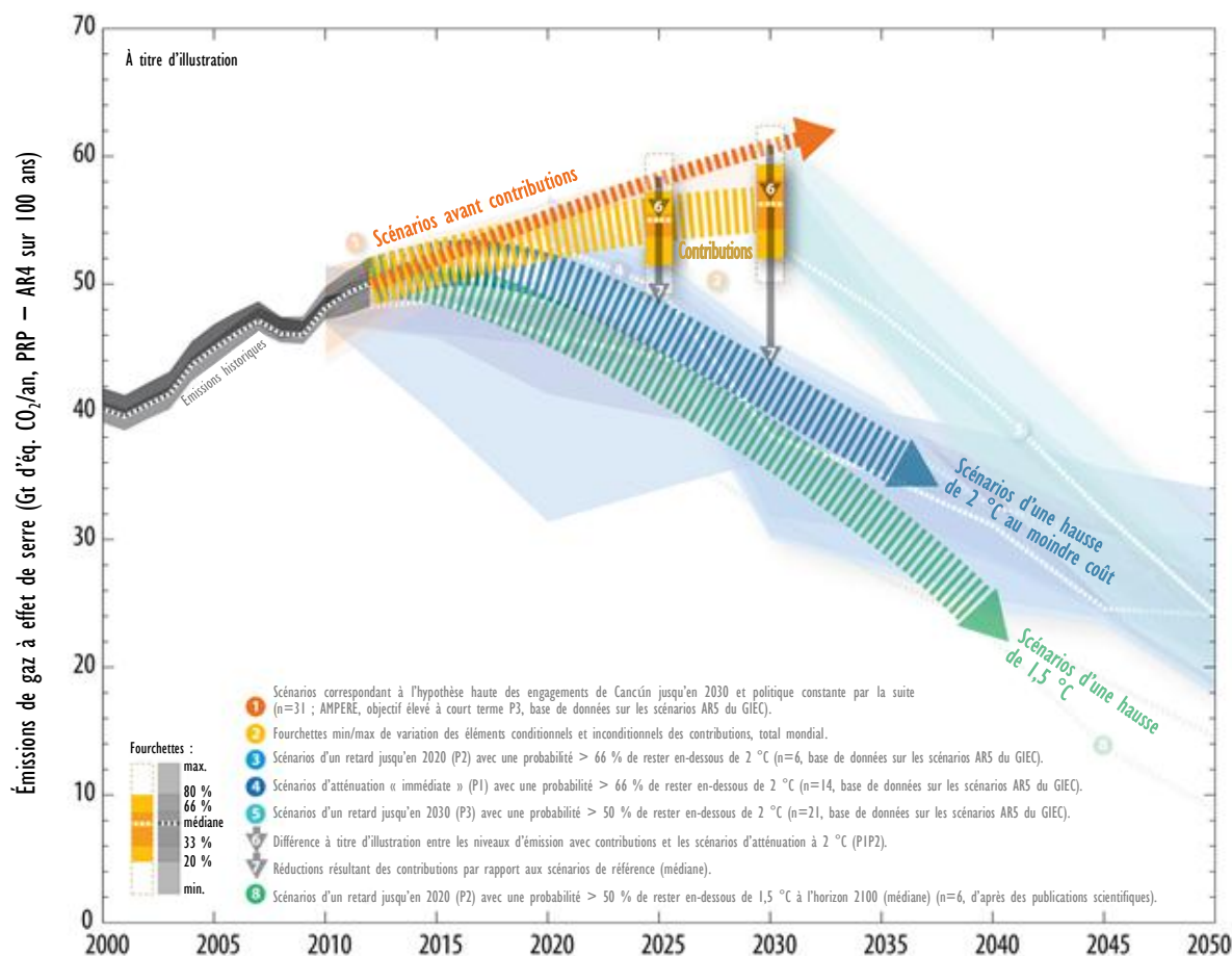
Figure 2 Comparaison des niveaux des émissions mondiales en 2025 et 2030 résultant de la mise en œuvre des contributions prévues déterminées au niveau national et selon d'autres scénarios
